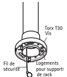
Support mural (exemple de fixation, vendu séparément)
