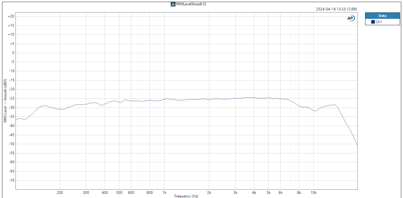
주파수 응답
